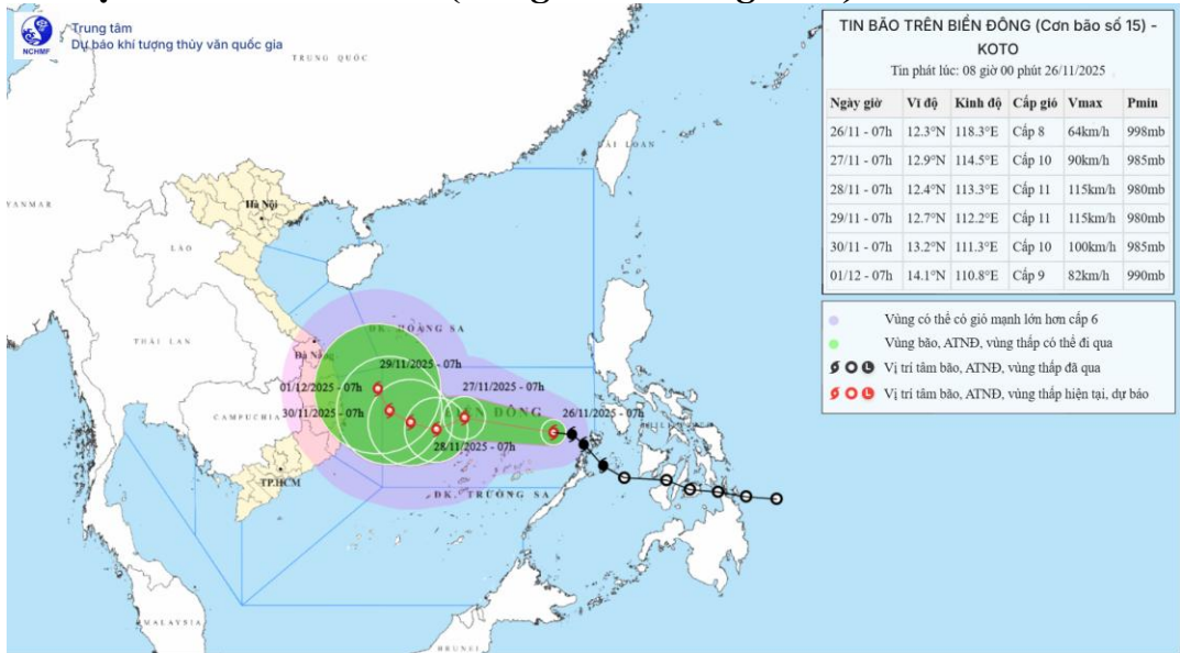
Hình 1. Bản đồ dự báo quỹ đạo và cường độ bão số 15 phát lúc 08h00 ngày 26/11/2025
